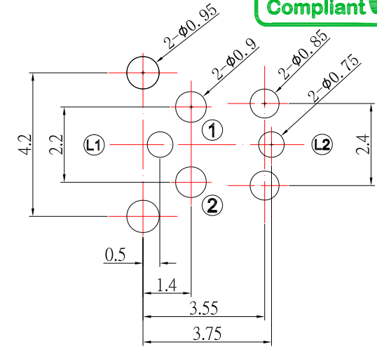
P.C.B LAYOUT
